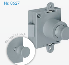
Fallen- und Drehstangenschloss, beidseitig bedienbar latch and espagnolette lock, operated from both sides Nr. 8627
