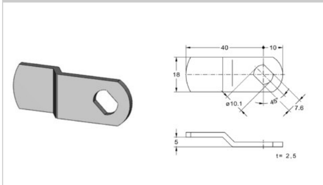
2642.401 Schließhebel
