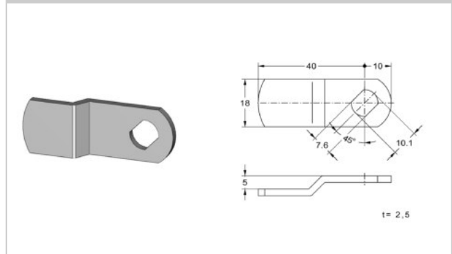
2642.402 Schließhebel
