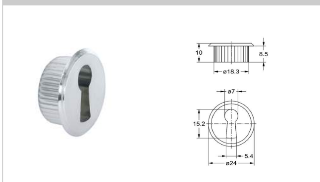
2103 Escutcheon
