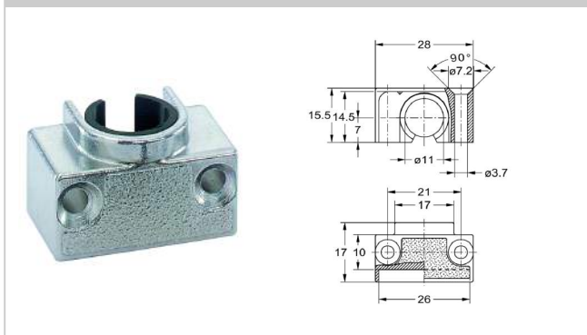
1319 Rod guide
