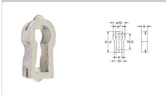
2104 Escutcheon
