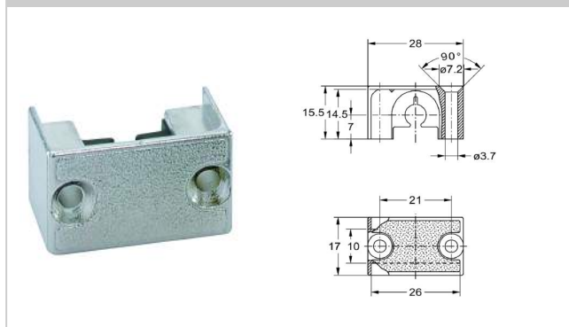
1318 Rod guide
